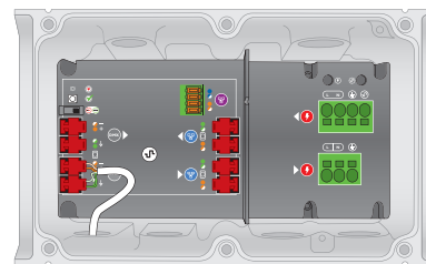
DMX input
